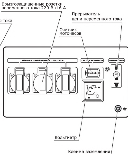
Рис. 10. Схема панели управления генератора УГД-5300 Basic
