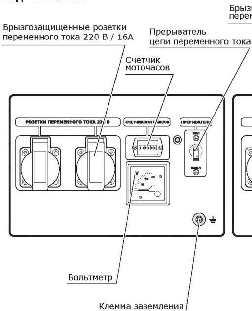
Рис. 9. Схема панели управления генераторов УГД-3000 Basic, УГД-4500 Basic
