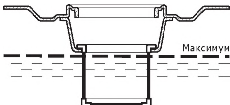
Рис. 13. Заполнение топливного бака и контроль уровня топлива
